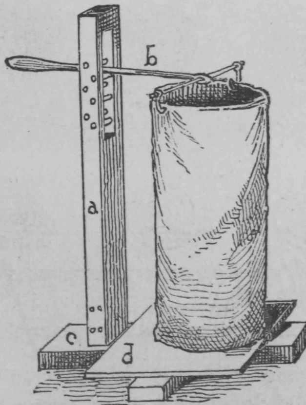
Fig. 163.—A HANDY BAG-HOLDER.
